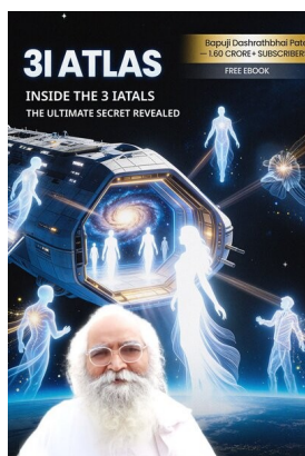
3i Atlas
