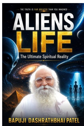
Aliens Life
